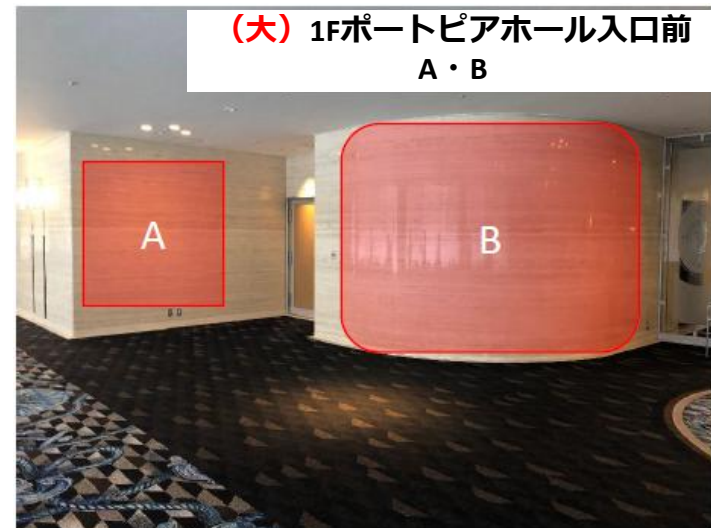
再剥離シート A:W2400×H2700 B:W5290×H2900
